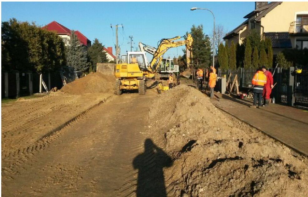
Zadanie rozbudowa sieci kanalizacji sanitarnej w Rogozinie w trakcie realizacji.
